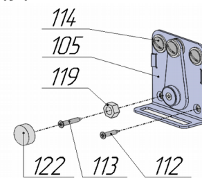
Рис.10.2 Закрепление при установке механизма на ПРАВОМ щите корпуса
